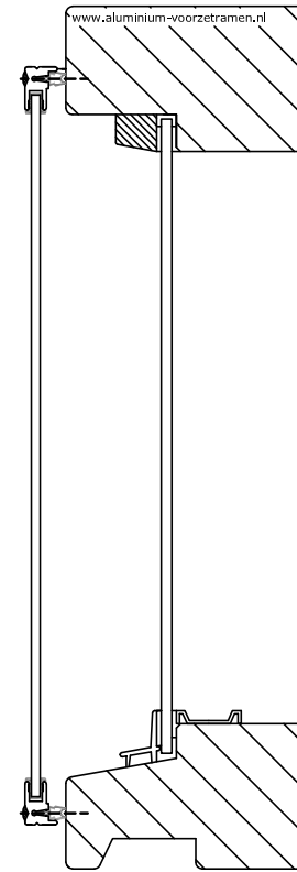
Montage voorzetraam met schroeven
