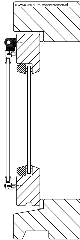
Montage voorzetraam met scharnieren en schroeven
