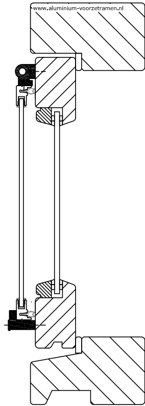
Montage voorzetraam met scharnieren en knevels
