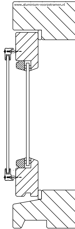
Montage voorzetraam met schroeven
