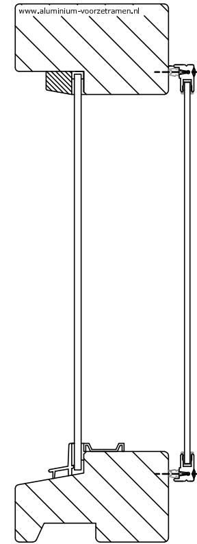
Montage achterzetraam met schroeven
